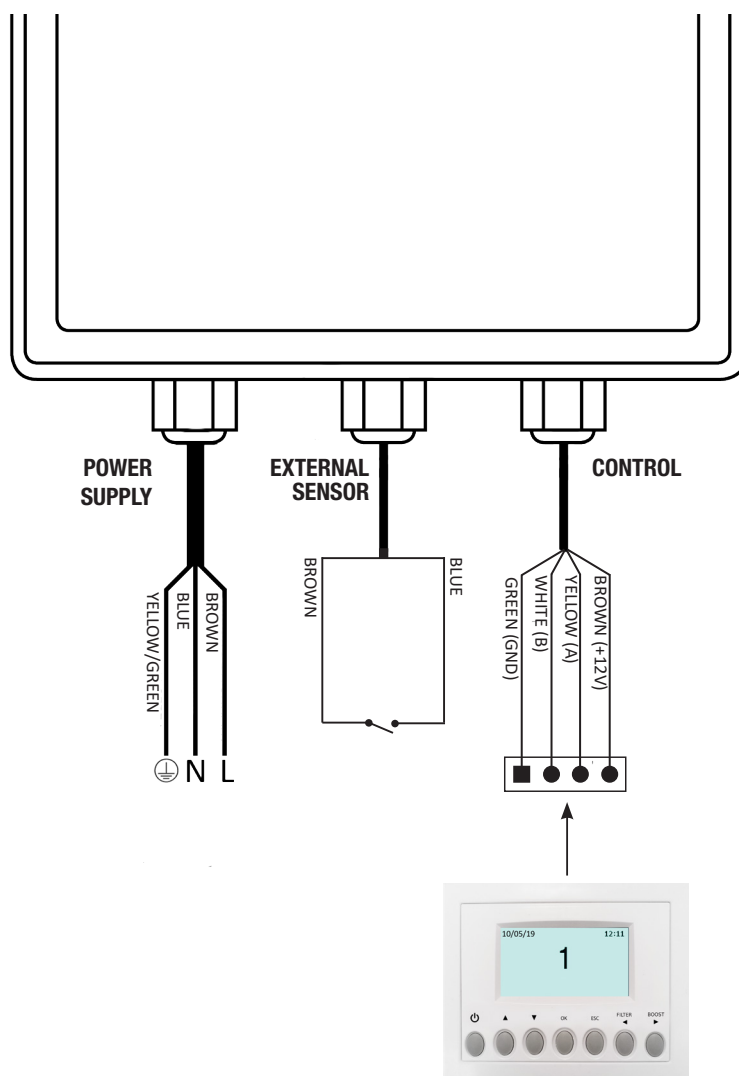
Fig. 5.f Precabling
