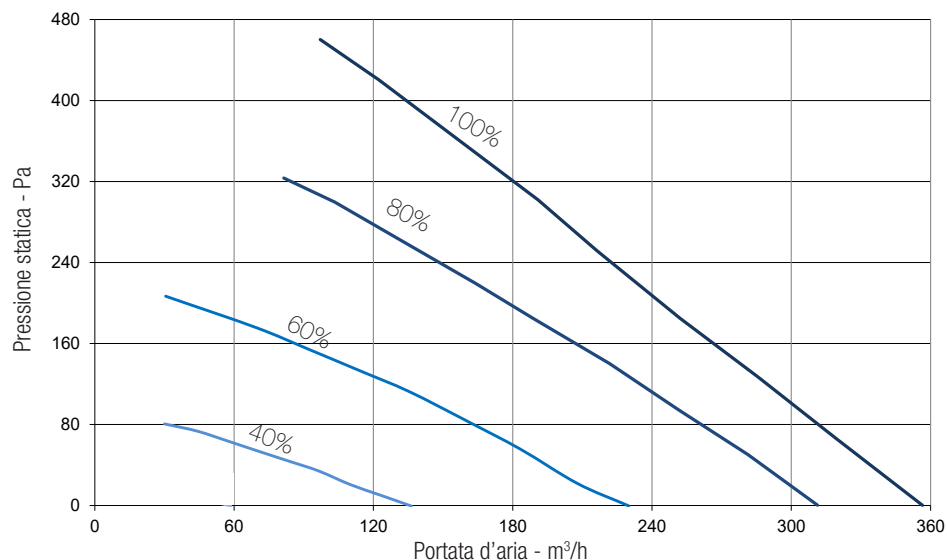
Fig. 6.c Curva di immissione in accordo al Reg. 1253/2014 (ErP).
