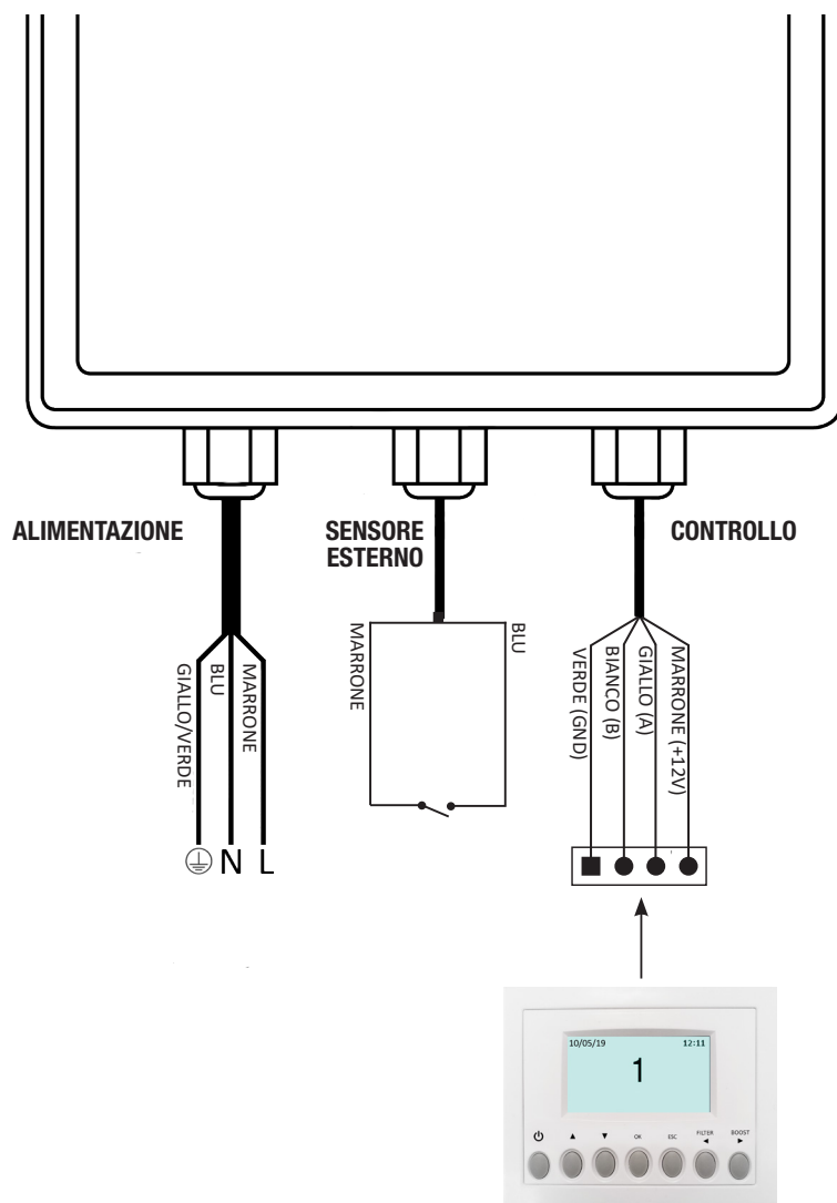
Fig. 4.f Precablaggio
