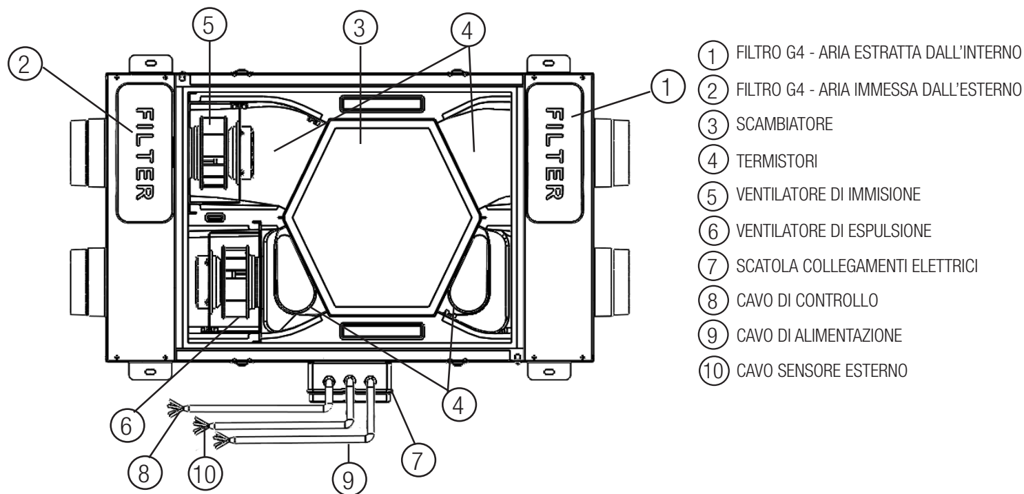
Fig. 7.a Componenti interni
